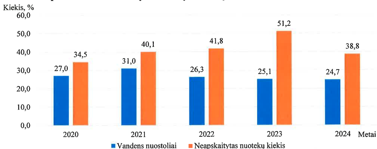
8 pav. Vandens nuostolių ir nuotekų infiltracijos kiekiai 2020-2024 m., proc.
